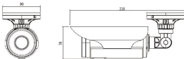
寸法図 (mm)
