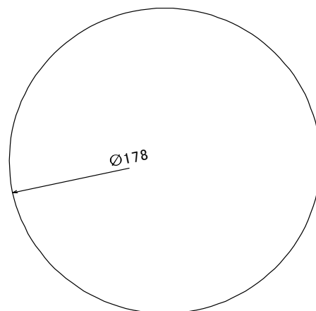
取り付け穴加工図
