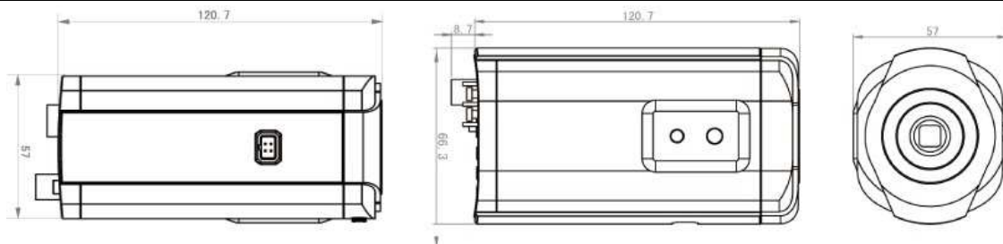
寸法図(mm)
