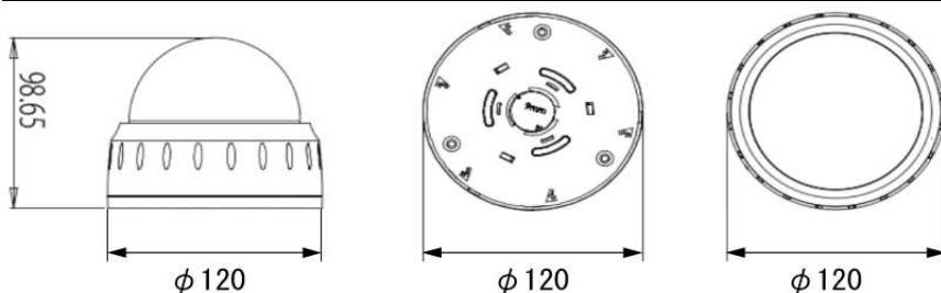
寸法図(mm)
