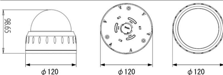
寸法図(mm)
