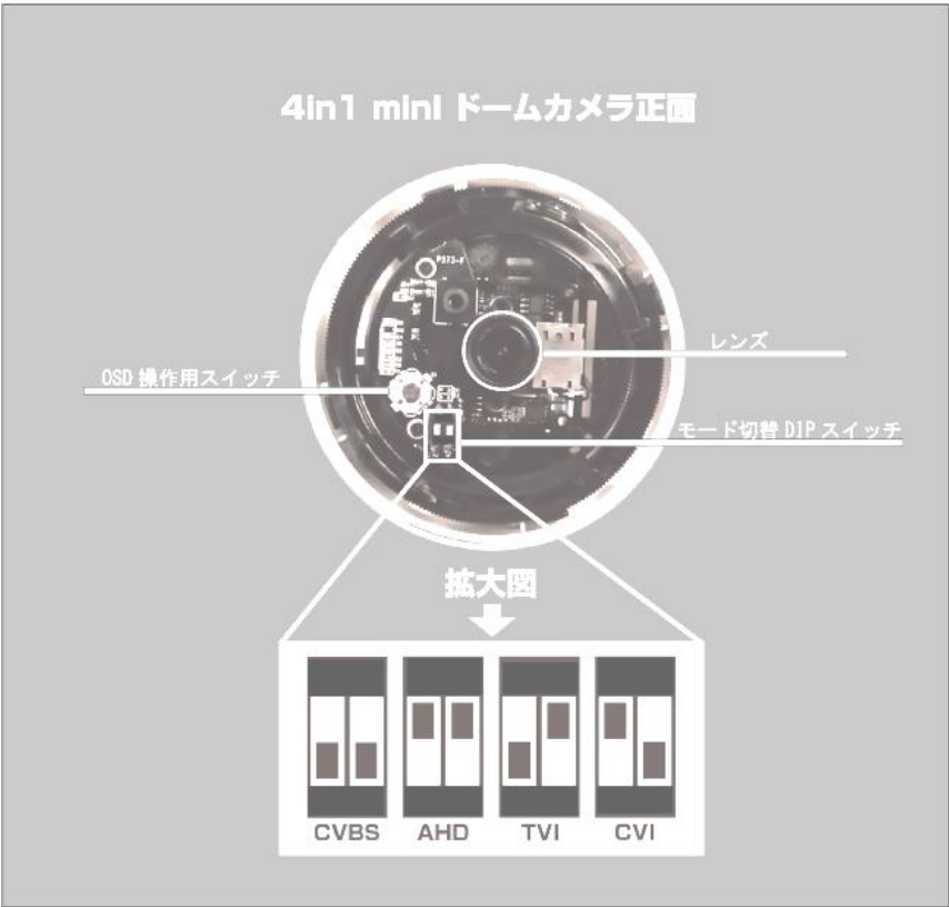
各映像モード、DIPスイッチ設定例
