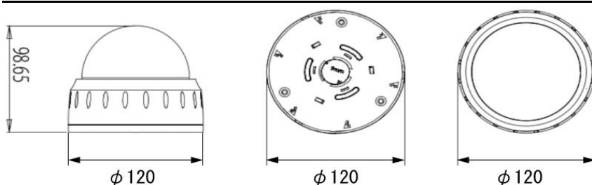
寸法図(mm)
