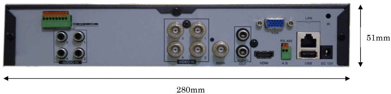
JV-465-UHJ (4ch) 外形寸法)
