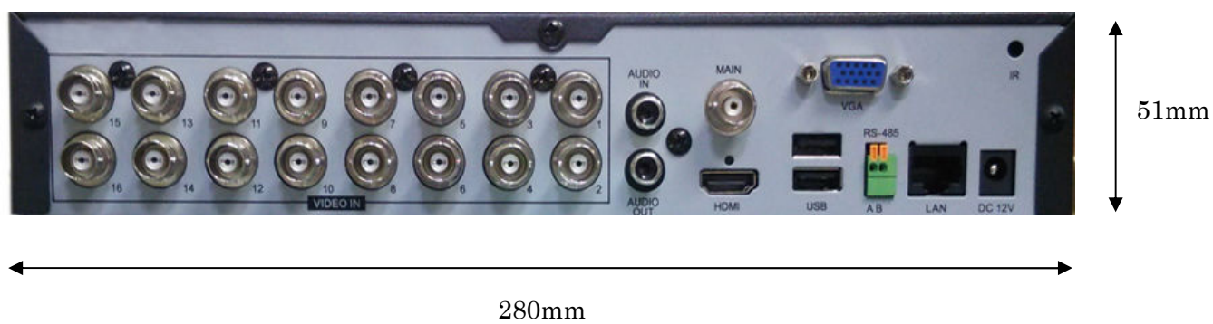
JV-1665-UHJ (16ch) 外形寸法)
