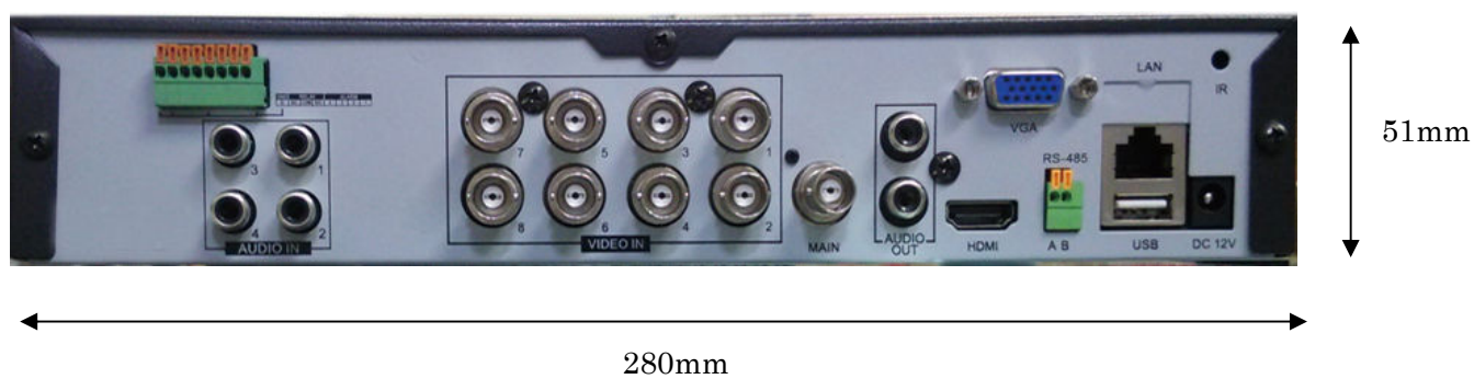
JV-865-UHJ (8ch) 外形寸法)
