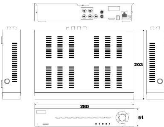
寸法図(mm)
